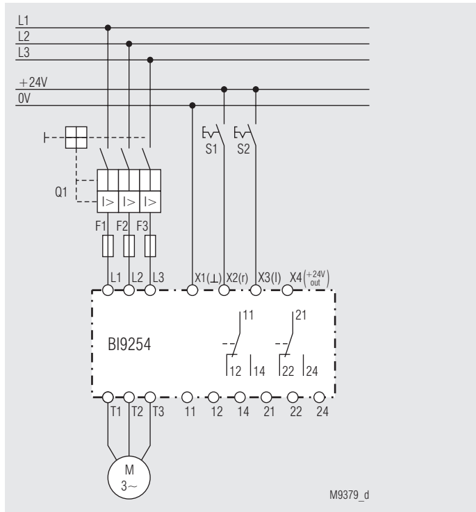
BI 9254 avec entrée de commande DC 24 V
