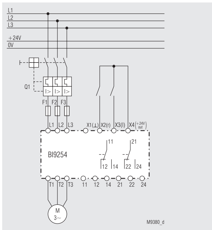
BI 9254 avec des contacts hors potentiel
