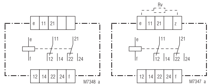
BA 9036 Anschlussbild für Wechselspannung
