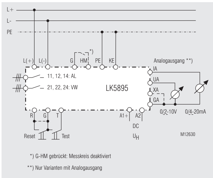
Isolationsüberwachung DC-seitig
