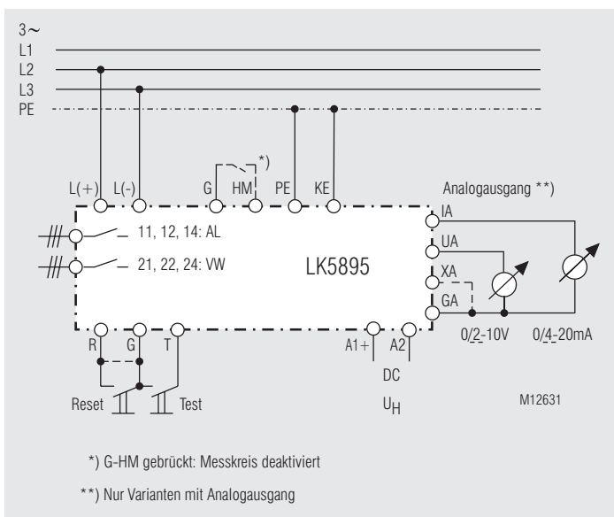
Isolationsüberwachung AC-seitig
