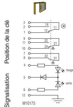
Fig. 2 : Verrouillage à l'état désactivé: 1 re Clé insérée (en bas) 2 e Clé à retirer (en haut)
