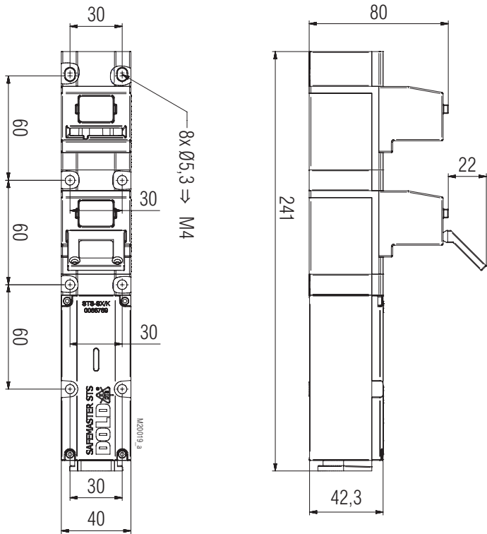
RX11M/K Freimaßtoleranzen \pm 2\%
